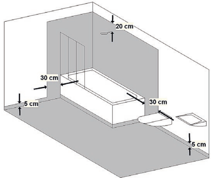
Abb. 2 Skizze zu Überständen der Badabdichtung gemäß Merkblatt 5 der Gipsindustrie
